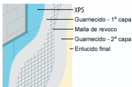
Figura 9. Detalles constructivos.
